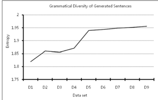
그림 9 생성된 문장의 엔트로피. 스탠포드 파서를 이용하여 생성된 문장의 문법 규칙을 찾은 후 문법 규칙의 복잡도를 엔트로피로 표현하였다. 생성된 문장의 엔트로피 분석을 통해 문법을 통해 문장 생성의 기반이 되는 하이퍼네트워크 모델의 복잡도가 높아졌음을 유추할 수 있다.
