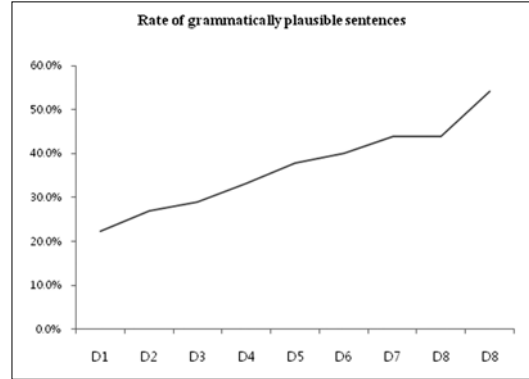
그림 8 문법적으로 성립하는 문장의 비율. 200개의 테스트 문장에 대하여 두 명의 평가자가 문법적 성립 여부를 평가한 결과, 두 명의 평가자가 문법적으로 성립 여부를 판정한 후 판정 결과의 평균치를 결과로 제시하였다.
