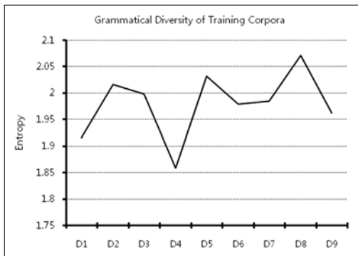
그림 4 훈련 코퍼스의 복잡도. 훈련용 코퍼스를 파싱한 후 파싱 트리의 문법 규칙 엔트로피로 복잡도를 계산
