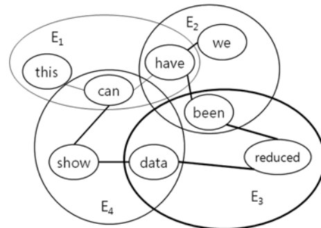
그림 1 하이퍼네트워크의 표현 예. 하이퍼네트워크 H = (X, E, W) 는 주어진 데이터 노드의 조합에 가중치를 부여한 항의 합으로 데이터의 분포를 표현한다.
