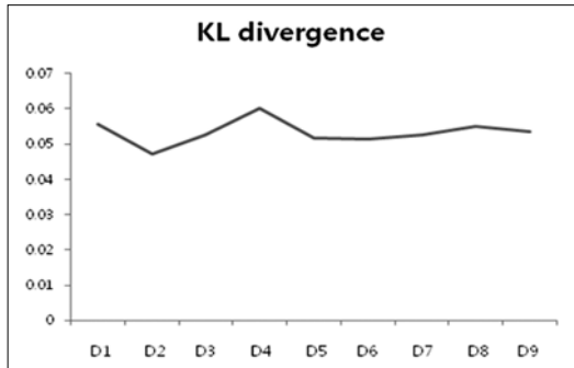
그림 10 학습 코퍼스의 문법 규칙 분포와 생성된 문장의 문법 규칙 분포 비교. 스탠포드 파서를 이용하여 획득한 문법 규칙의 분포에 대하여 KL 다이버전스를 계산한 결과
