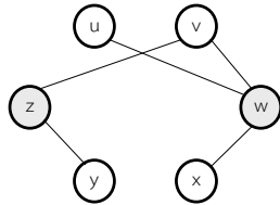
กราฟ G' มี VC ขนาด 2
