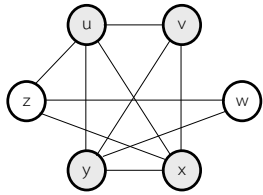
กราฟ G มี clique ขนาด 4
